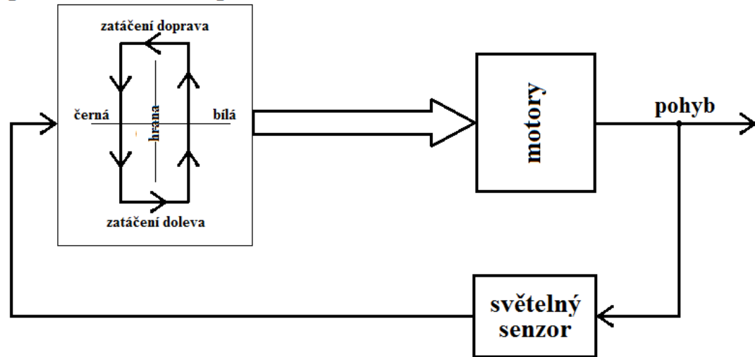
regulátor (cik-cak algoritmus)
