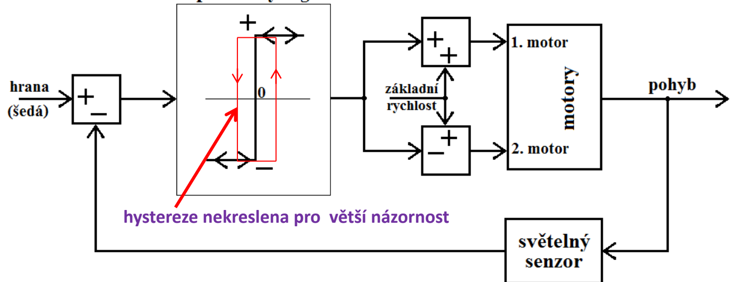
dvoupolohový regulátor
